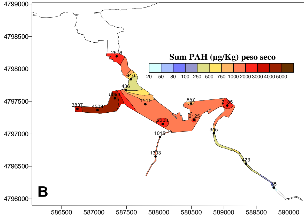
Figura 5.10 : Distribución del sumatorio de valores de PCB (a) y del sumatorio de valores de PAH (b) en los sedimentos del río Oiartzun y de la bahía de Pasaia.
