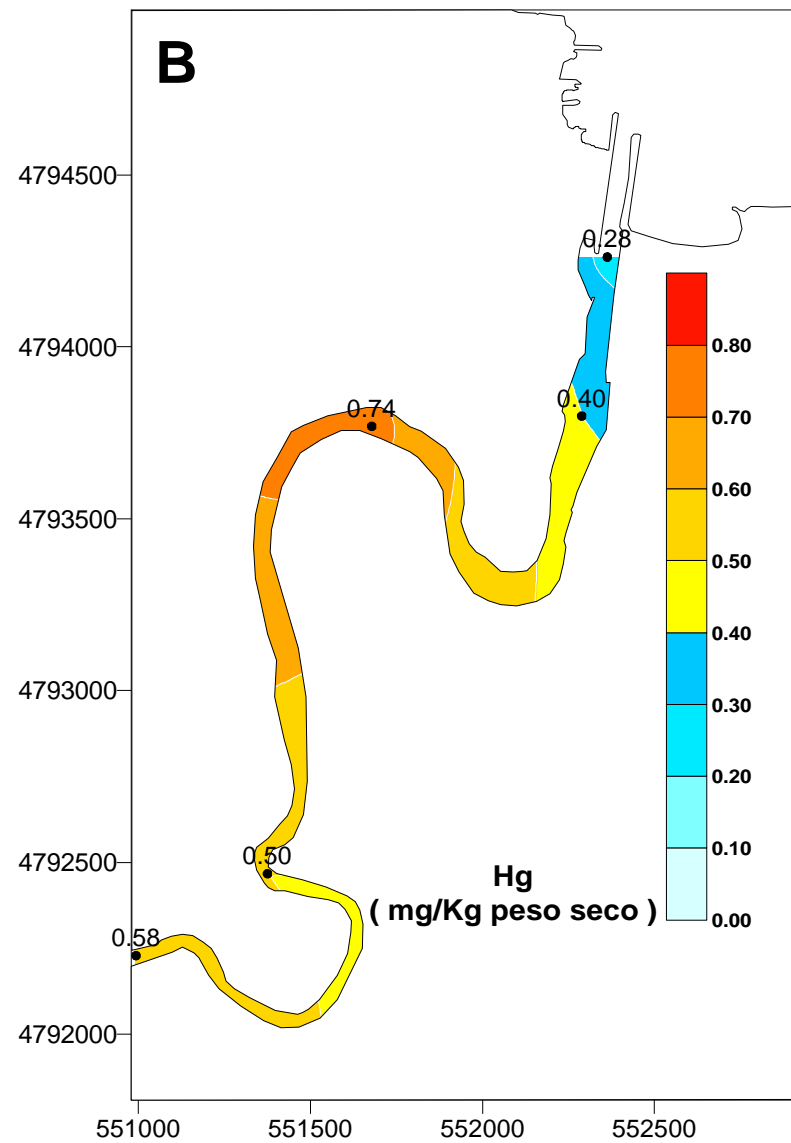
Figura 7.6 : Distribución de los valores de cobre (a) y mercurio (b) en los sedimentos del río Deba.
