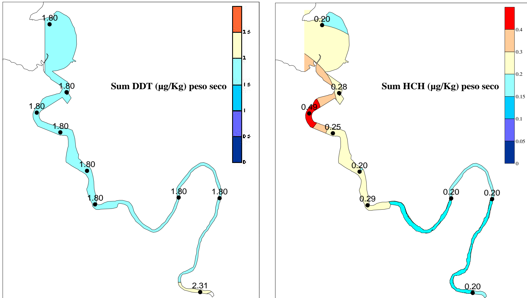
Figura 6.11. Distribución del contenido de DDT y HCH en los sedimentos del estuario del Butroi.
