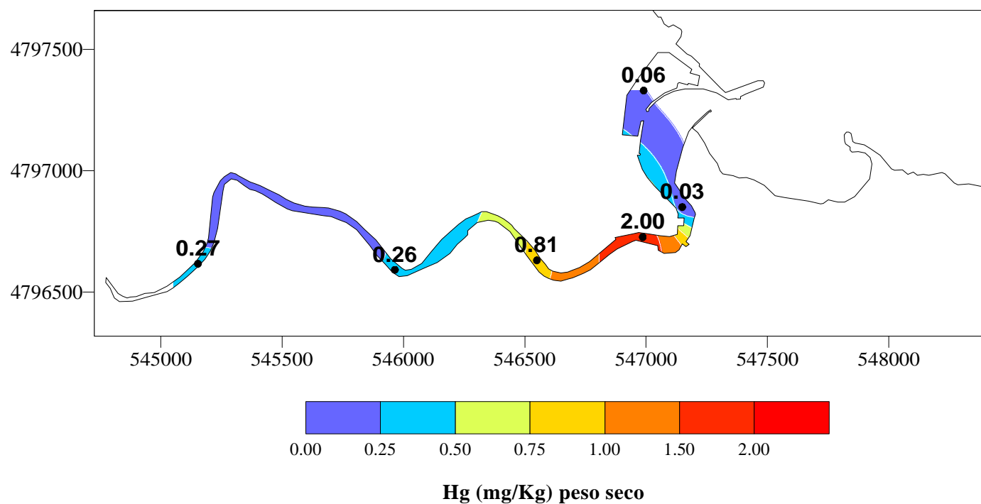
Figura 7.6. Distribución del contenido de arsénico y mercurio en los sedimentos del estuario del Artibai.
