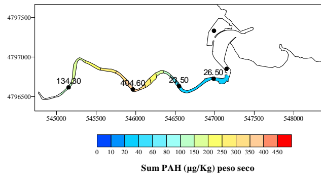
Figura 7.10. Distribución del contenido de PCB y PAH en los sedimentos del estuario del Artibai.
